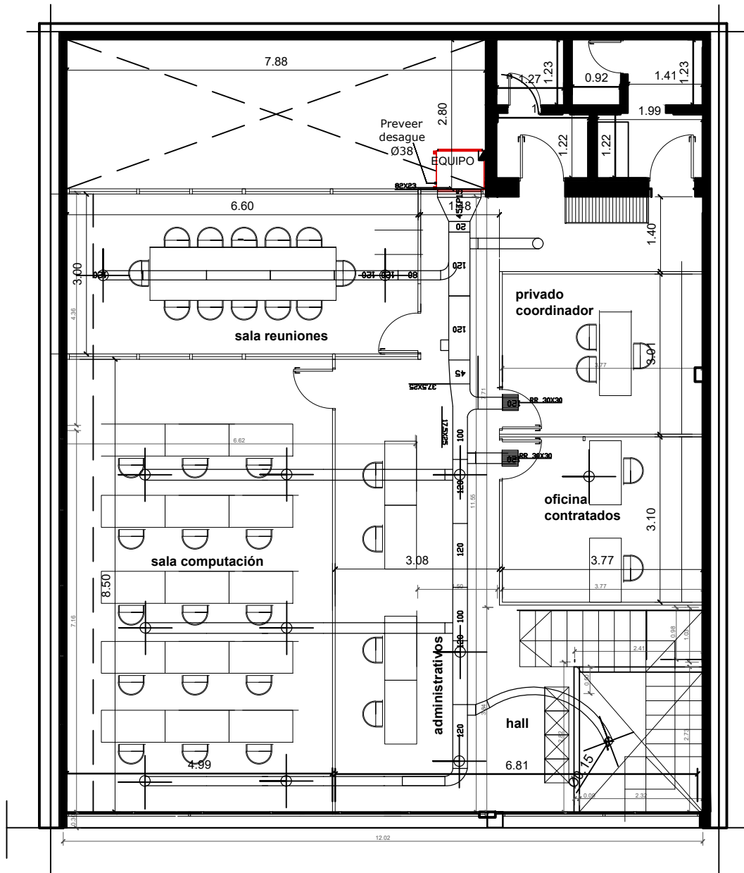
PLANTA ALTA INSTALACIÓN EQUIPO CENTRAL FRÍO CALOR
