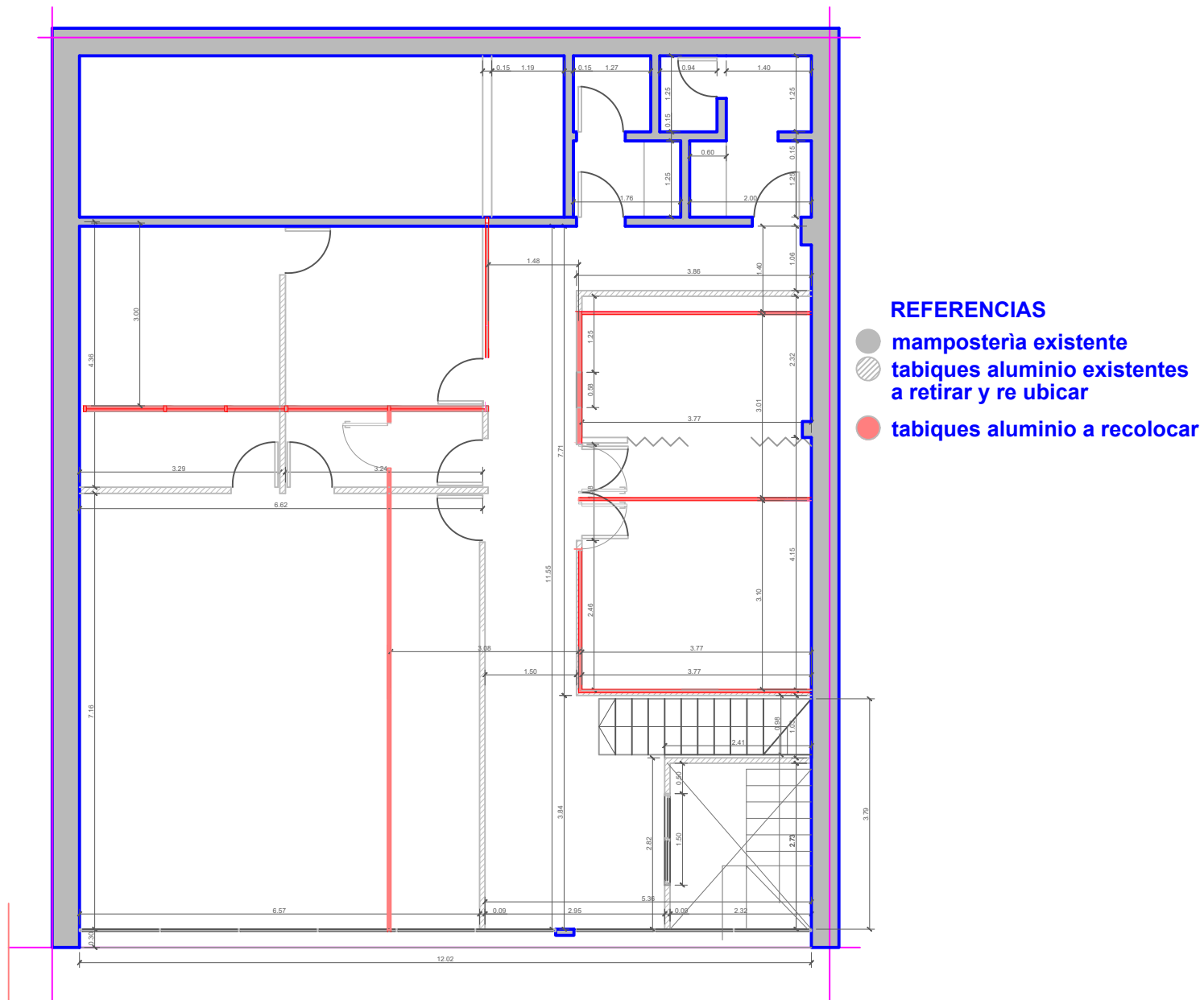
PLANTA ALTA
